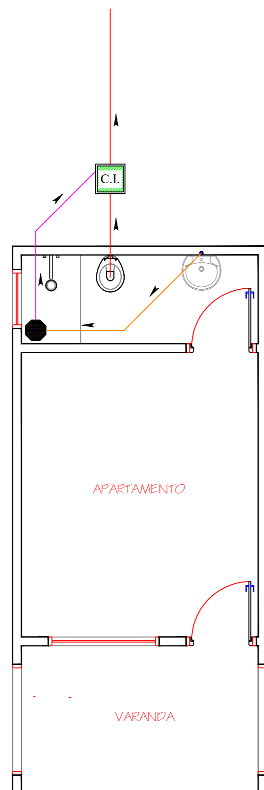
Planta Baixa Esgoto ESCALA 1/50
