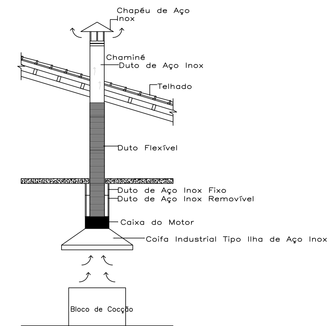
2 DETALHE DA TUBULAÇÃO DE EXAUSTÃO ESC: 1:50
