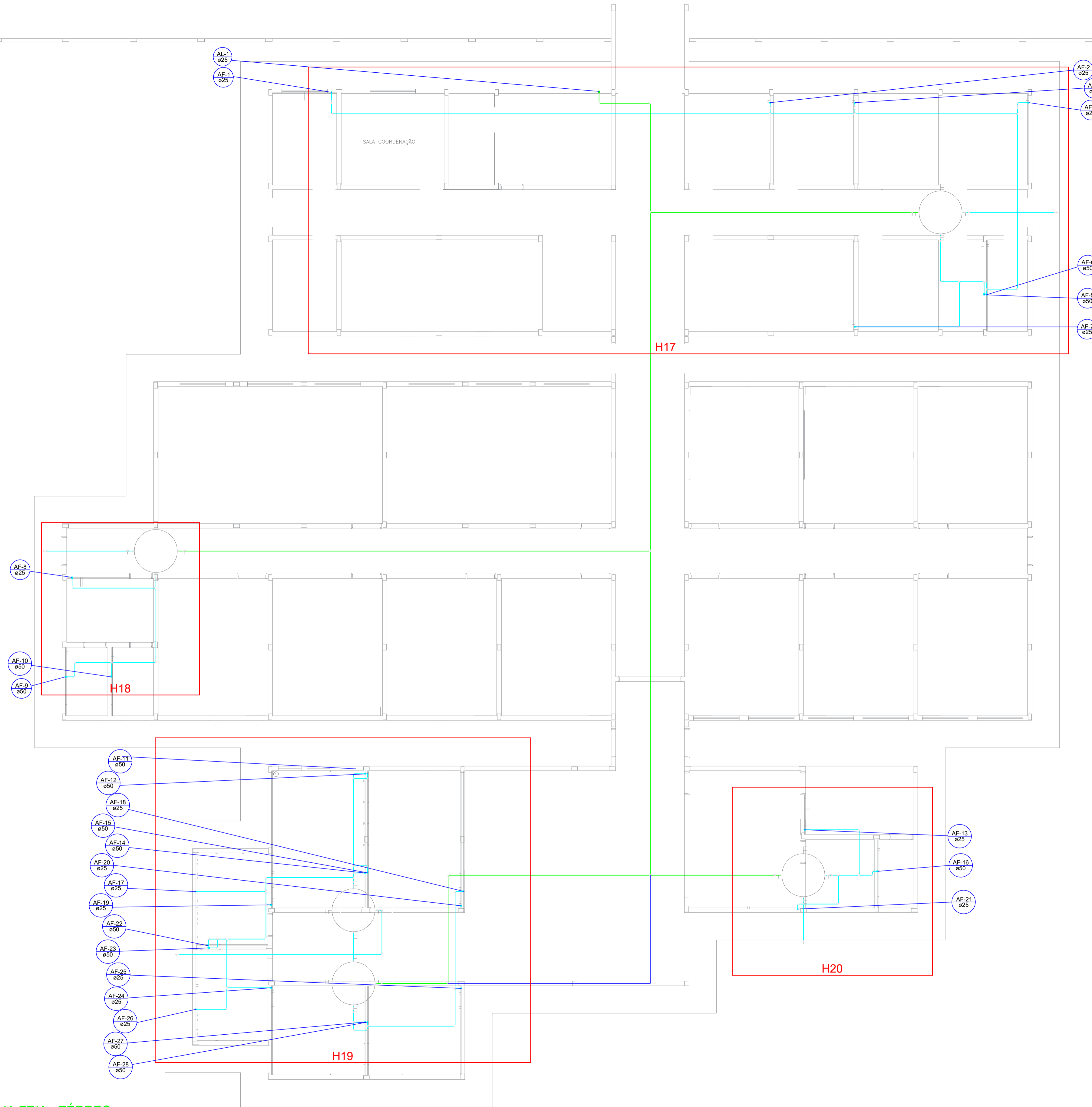
PLANTA ÁGUA FRIA - TÉRREO esc 1:100
