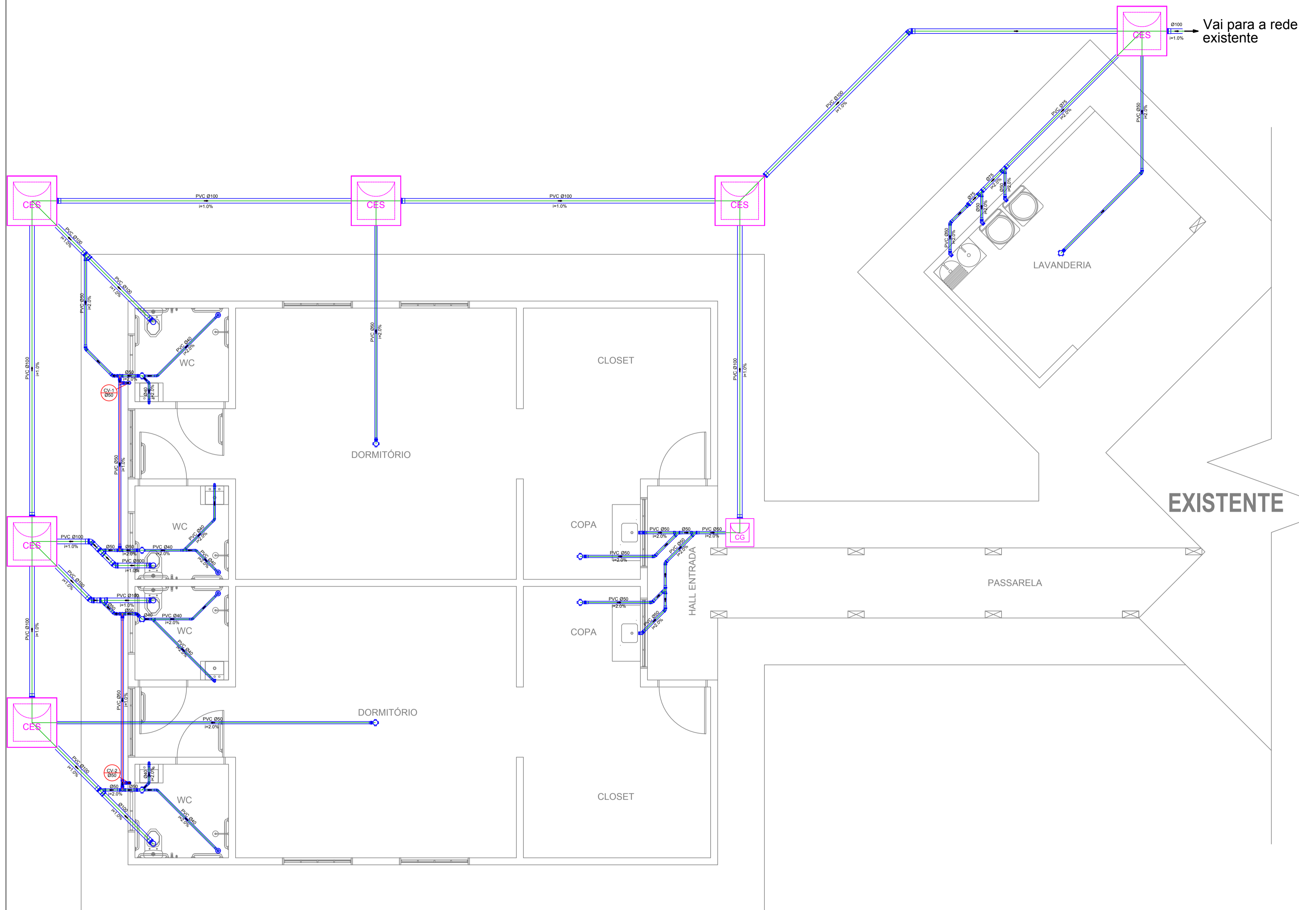
PLANTA BAIXA Escala 1:50
