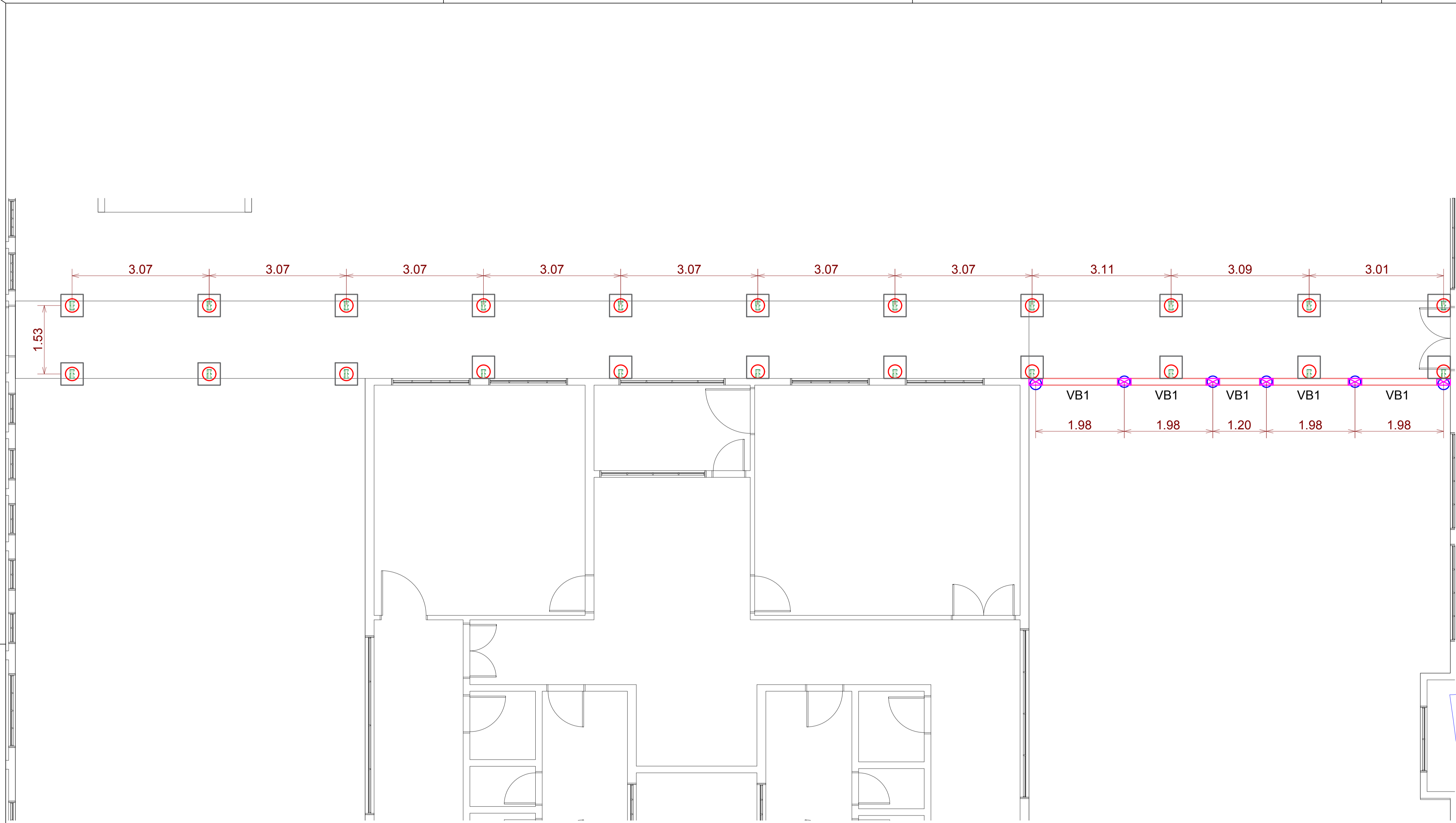
LOCAÇÃO DAS BROCAS, BLOCOS, VIGAS BALDRAMES E PILARES - PASSARELA ESCALA 1/50
