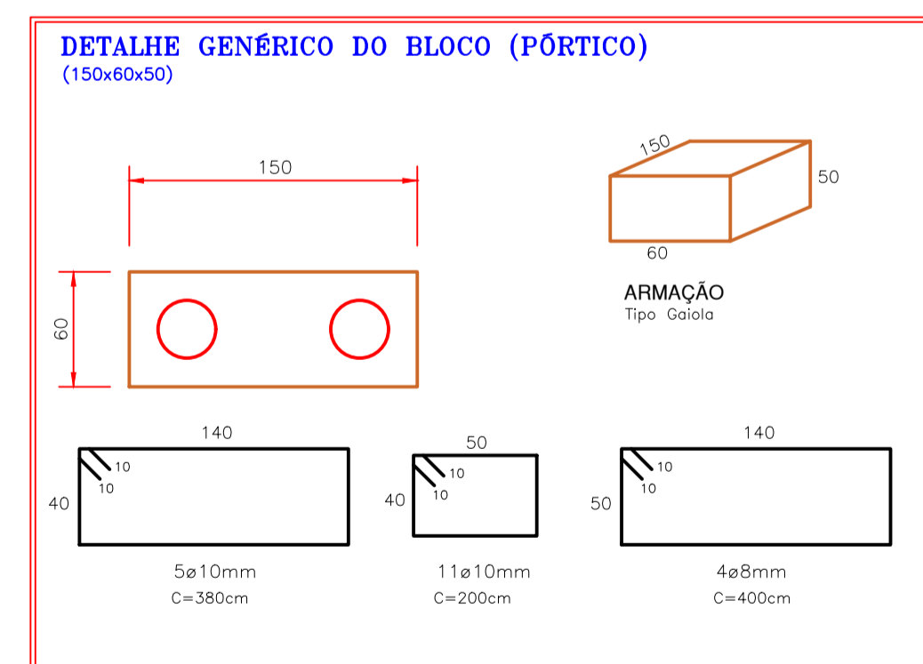
DETALHES DAS BROCAS, BLOCOS, VIGAS BALDRAMES E PILARES SEM ESCALA
