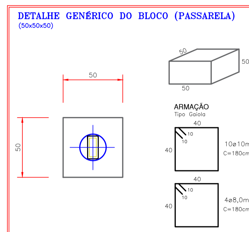
DETALHES DAS BROCAS, BLOCOS, VIGAS BALDRAMES E PILARES SEM ESCALA
