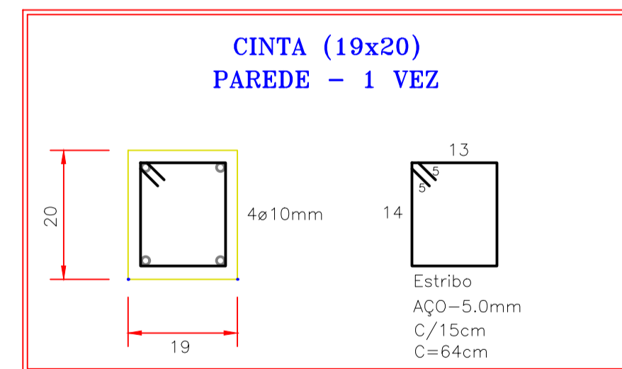
DETALHES PILARES, VERGAS, CONTRAVERGAS E CINTAS SEM ESCALA
