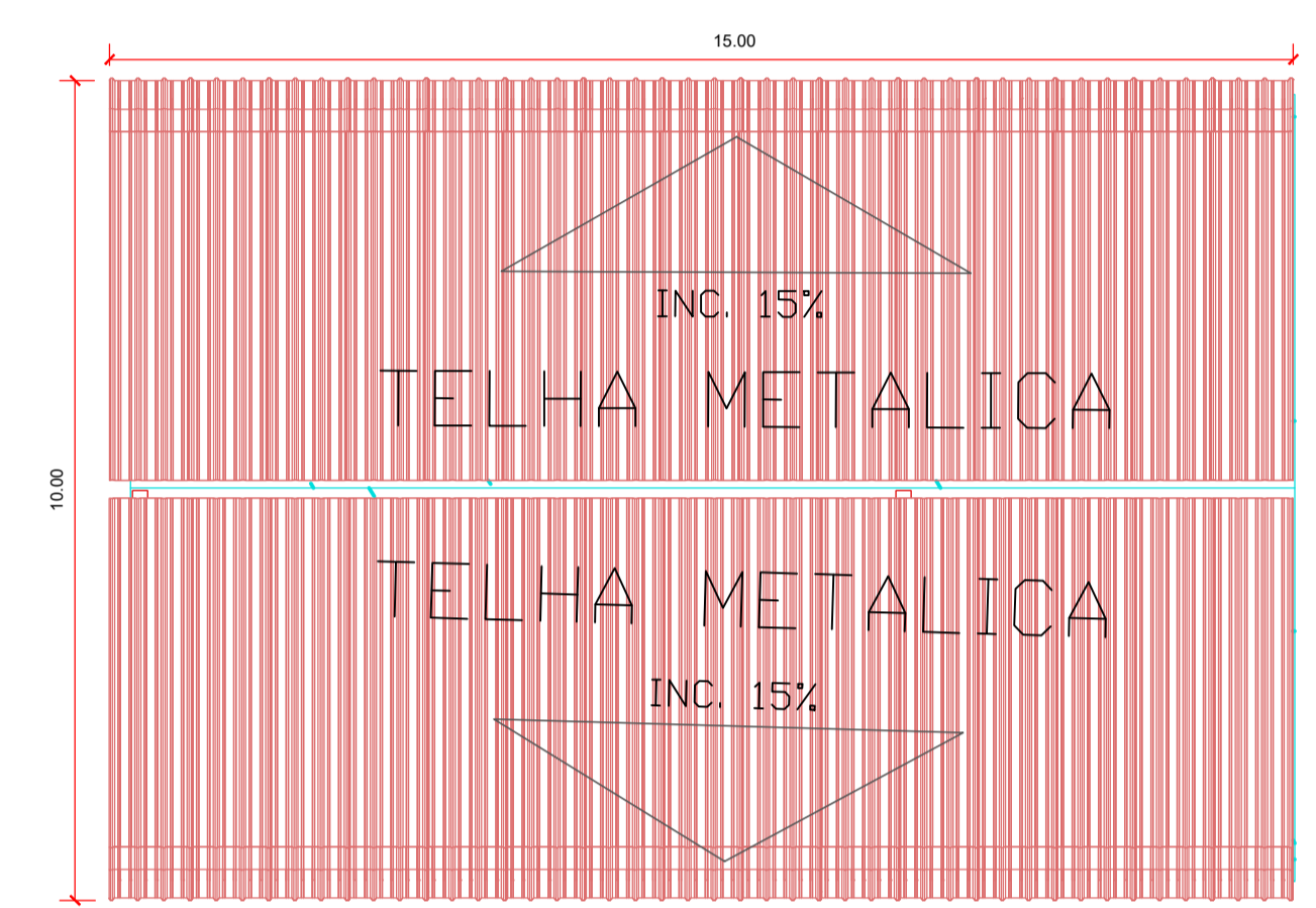
PREDIO CALDEIRA - COBERTURA ESC.: 1/50
