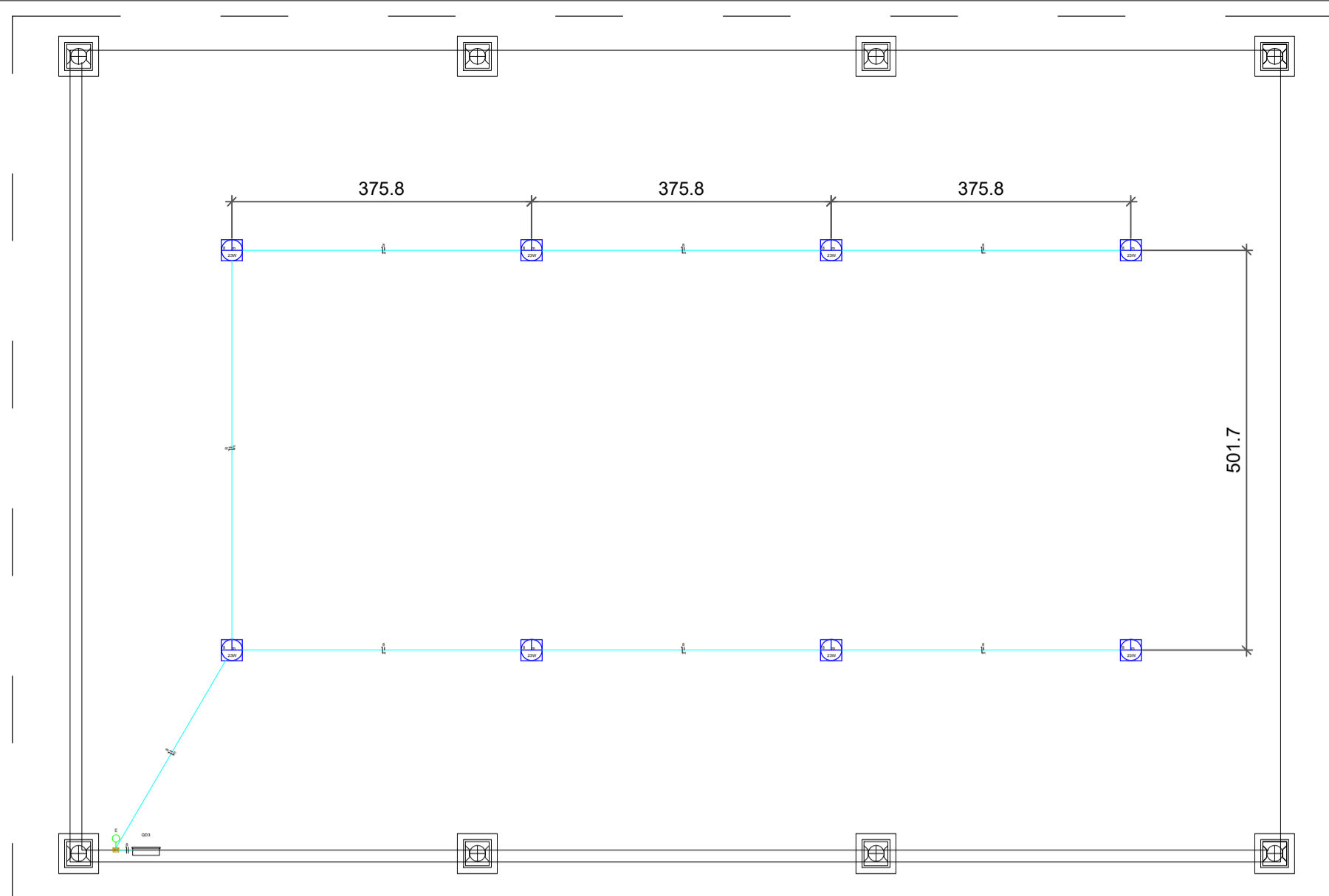
Detalhe D3 Escala 1:70
