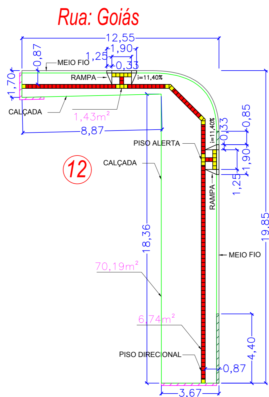
PLANTA BAIXA ESC 1/75
