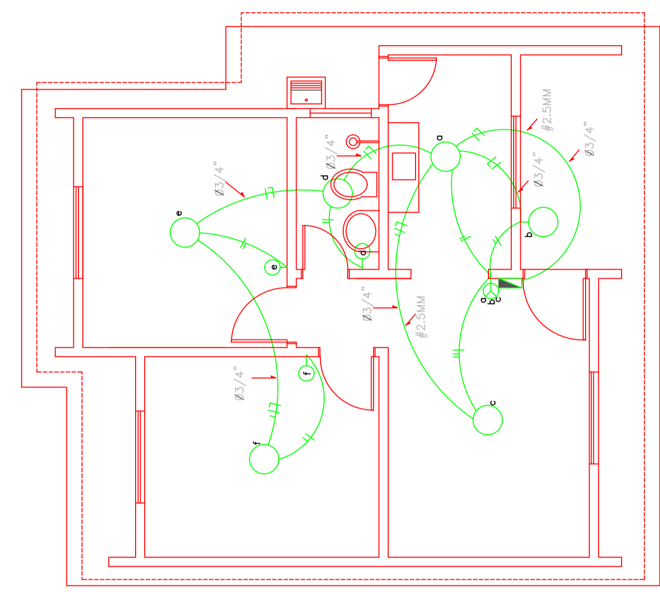
02 PROJETO ELÉTRICO - ILUMINAÇÃO CASA 2 DORMITÓRIOS A= 41,16 m² Esc.:1:50
