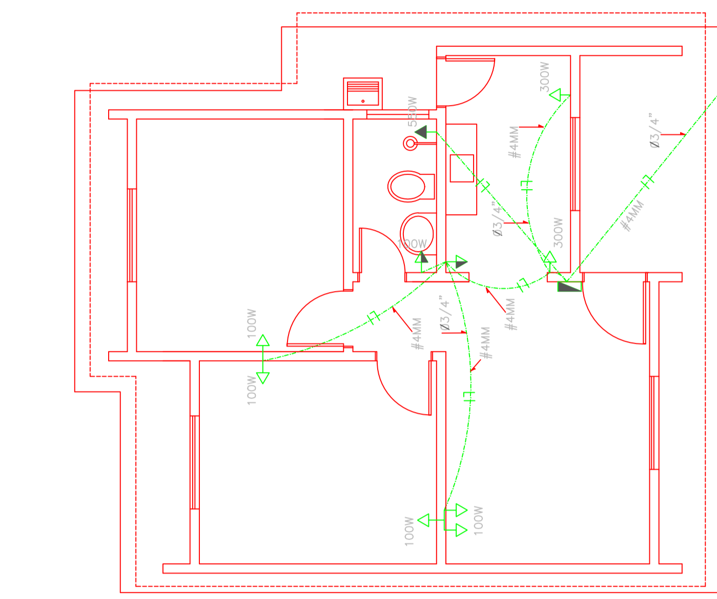
01 PROJETO ELÉTRICO - FORÇA CASA 2 DORMITÓRIOS A= 41,16 m² Esc.:1:50
