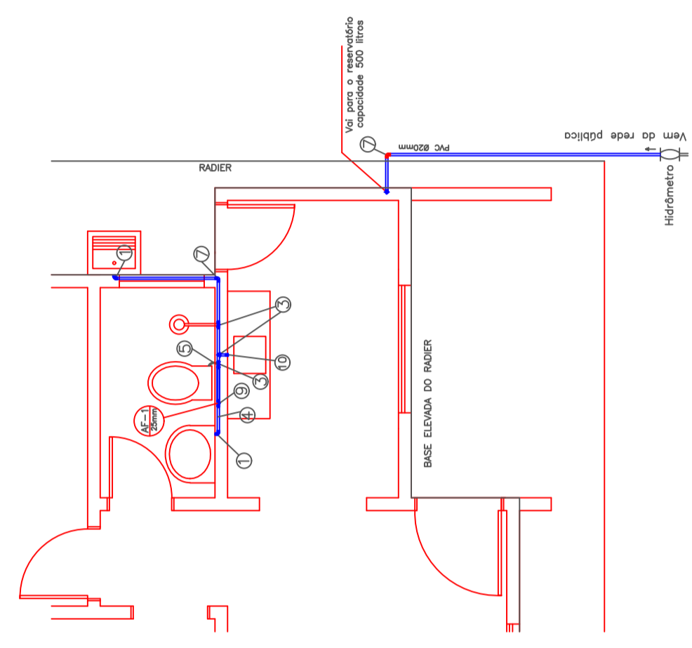
03 PROJETO HIDRÁULICO CASA 2 DORMITÓRIOS A= 41,16 m² Esc.:1:50
