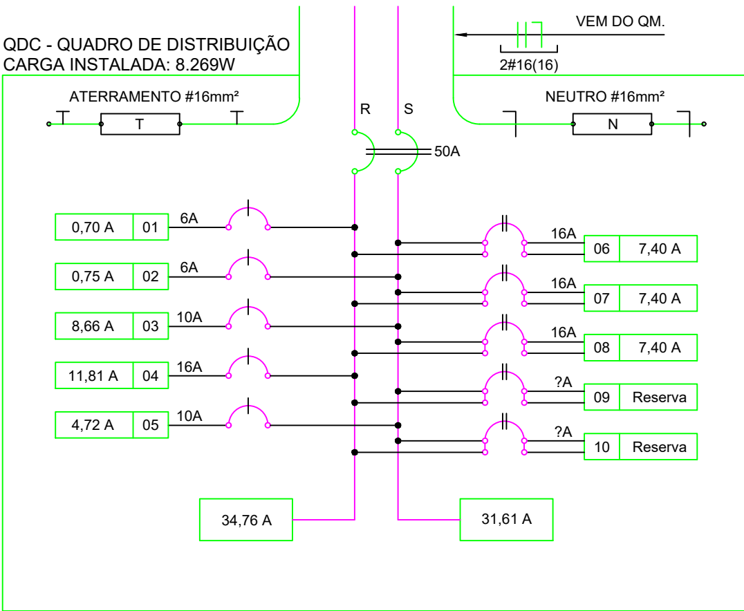
1 DIAGRAMA MULTIFILAR - QDC ESCALA: 1/50
