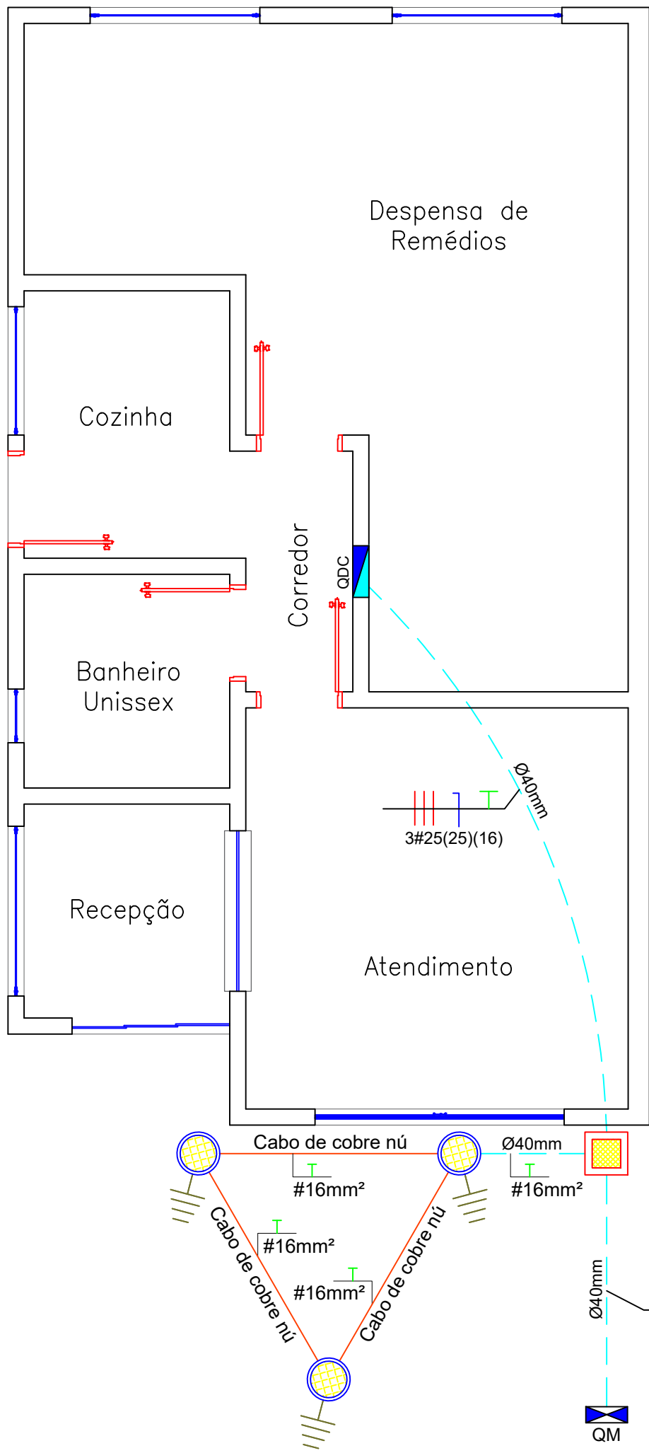
Aterramento ESCALA 1/50
