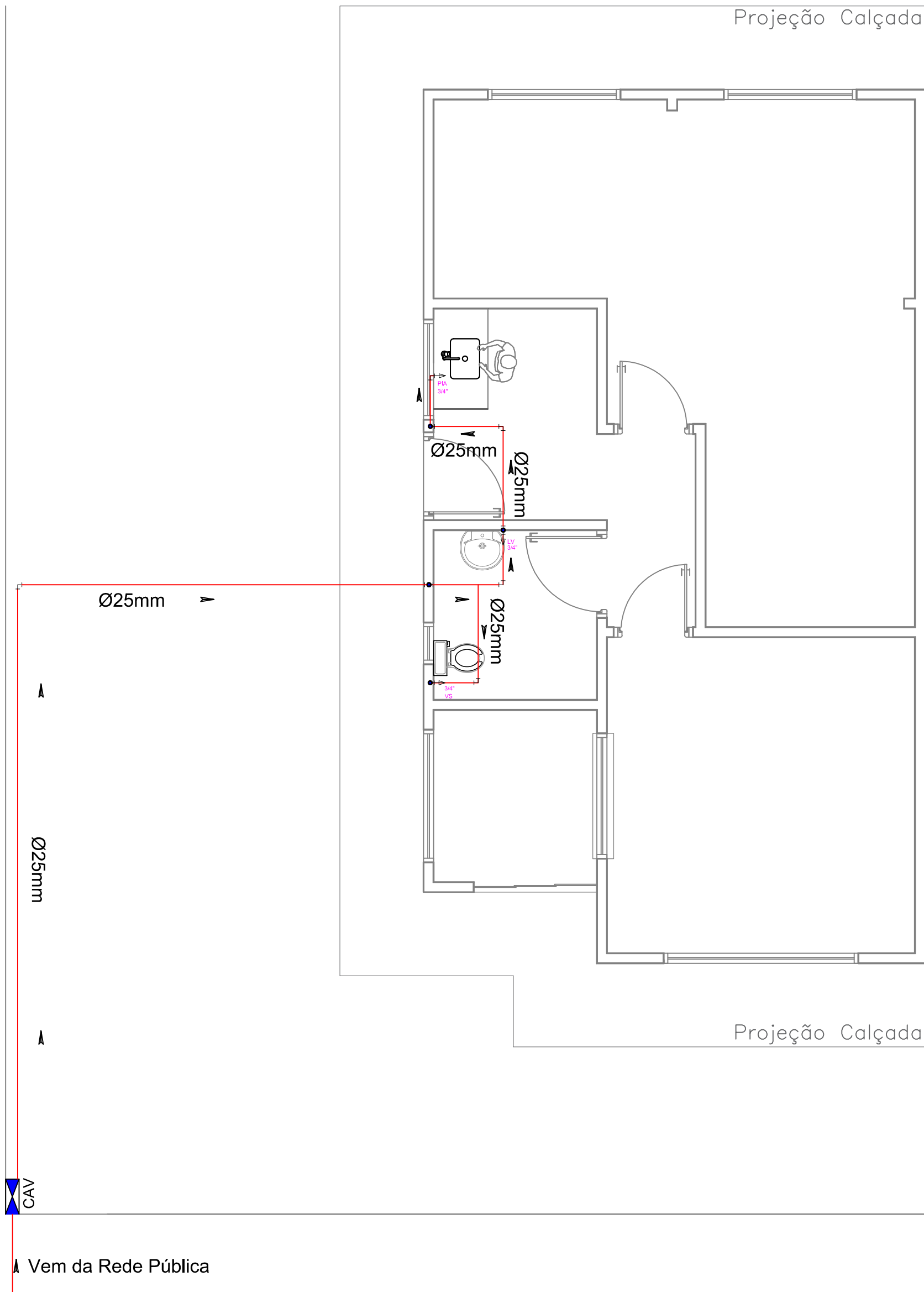
Planta Baixa - Rede de Água Fria ESCALA 1/50
