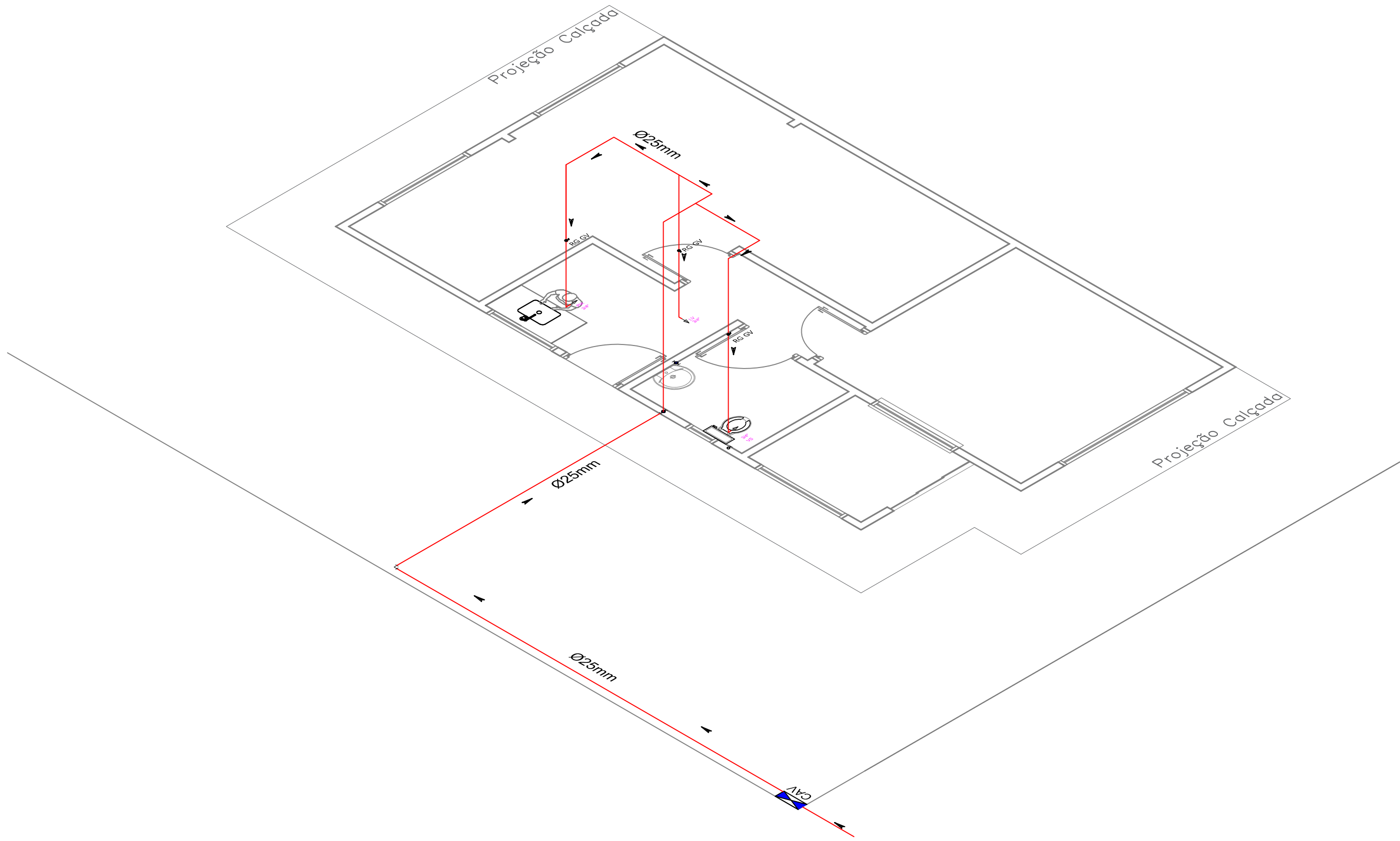
Planta Baixa - Isométrico ESCALA 1/50
