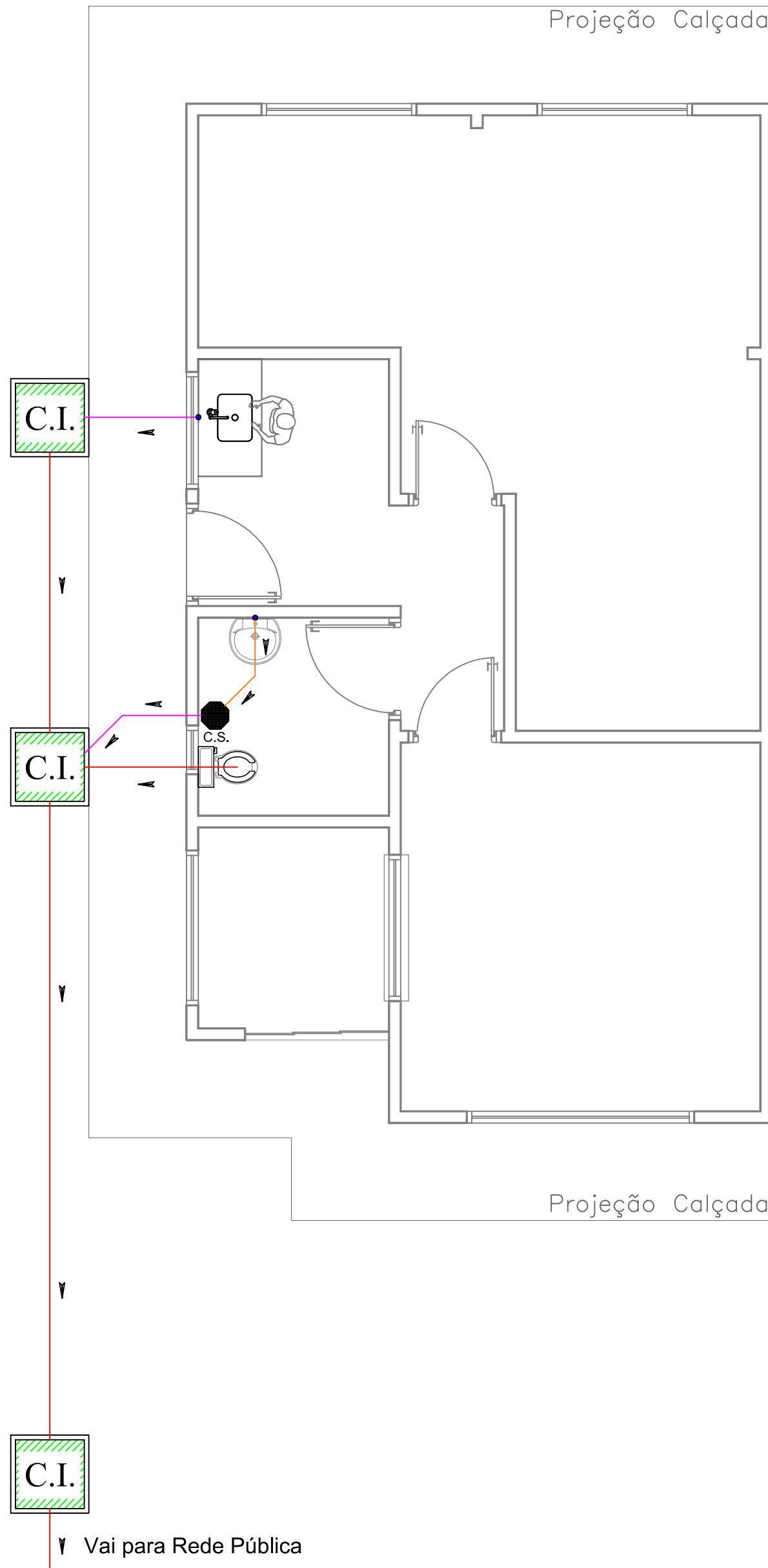
Planta Baixa - Rede de Esgoto Cloacal ESCALA 1/50
