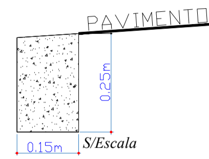
Detalhe do Tento de Concreto
