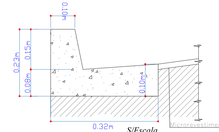
DETALHAMENTO DA SARJETA
