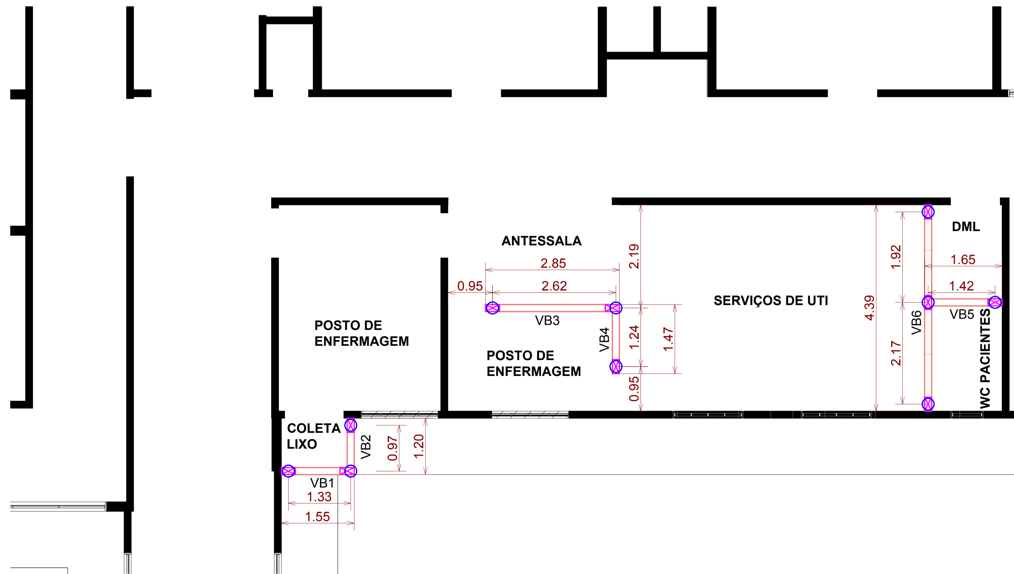
LOCAÇÃO DAS BROCAS, VIGAS BALDRAMES E PILARES - BLOCO 2 ESCALA 1/50
